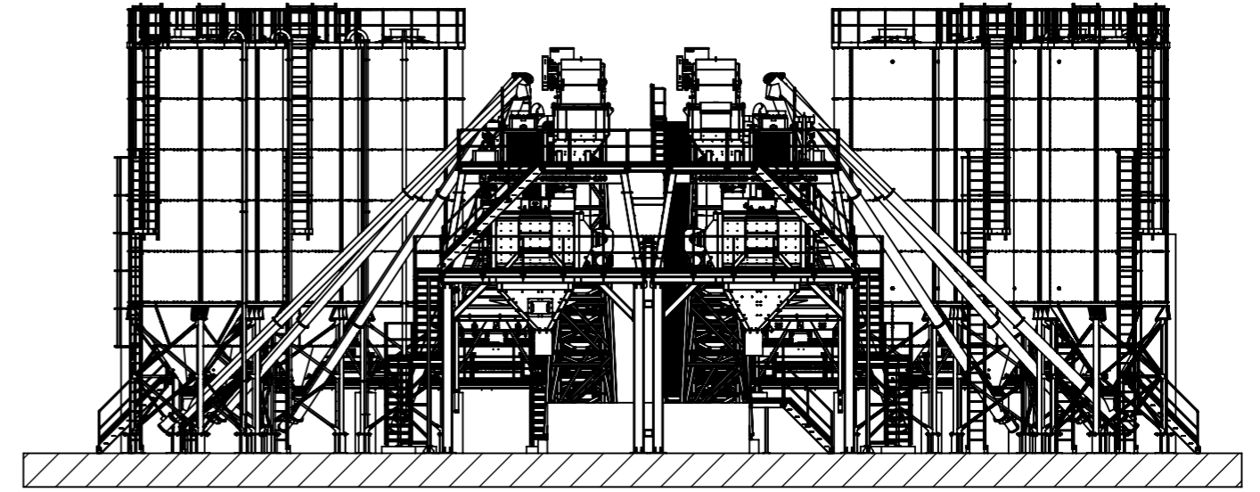
KESIT B-B
